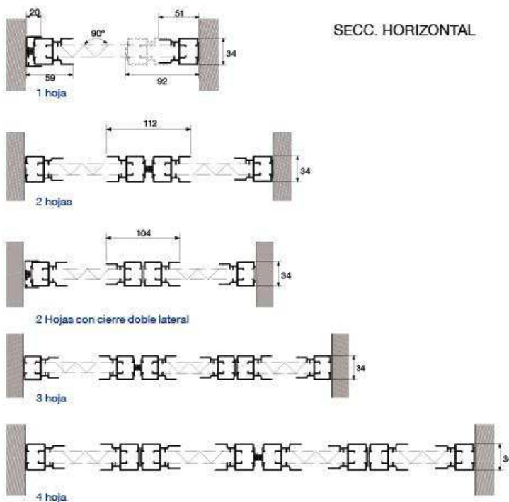
CONFIGURACIÓN 4 HOJAS
