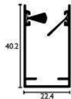
Gua Semi-Antiviento
