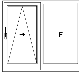
Esquema A – con travesaño central 1 hoja corredera, 1 hoja fija Dibujó: montaje mano izquierda
