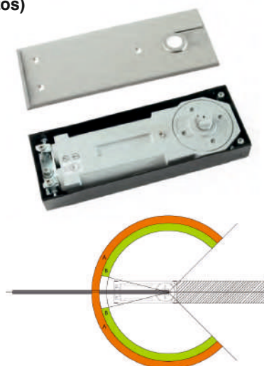
A - Rango primario de ajuste 130° a 0° B - Rango secundario de ajuste 130° a 20°
