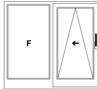
Esquema A – con travesaño central 1 hoja corredera, 1 hoja fija Dibujó: montaje mano derecha
