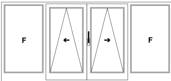
Esquema C – con travesaños centrales 2 hojas correderas, 2 hojas fijas Dibujó: Hoja de primera apertura con posición de manilla izquierda
