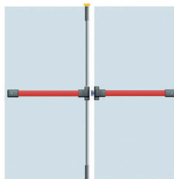
ESCAPE 4 Y ESCAPE 1 Antipánico 2 hojas Cierre superior e inferior + Cierre lateral.
