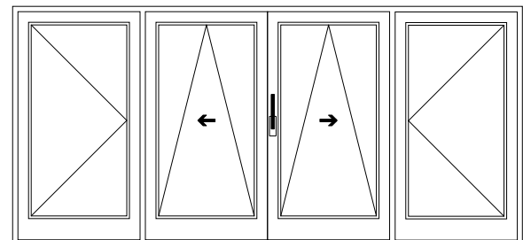
Esquema C – con travesaños centrales 2 hojas correderas, 2 hojas practicables Dibujó: Hoja de primera apertura con posición de manilla izquierda
